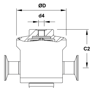
Optional dome-loading
