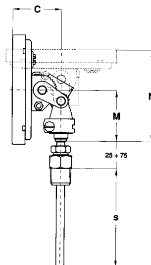
Montaggio snodato (Codice 2)
