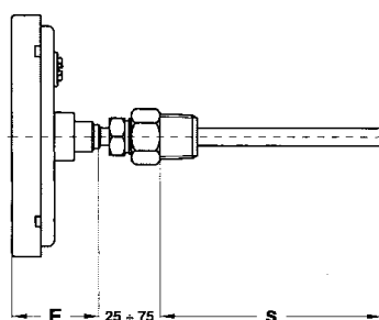
Montaggio posteriore (Codice 1)
